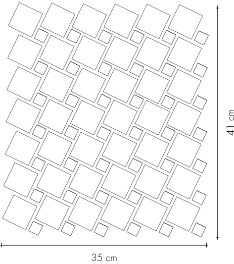
Quadrato 5x5 cm (2"x2") Tozzetto 2x2 (3/4"x3/4") cm
