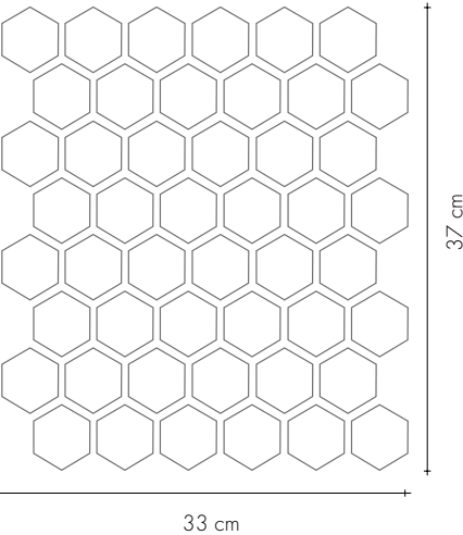
Esagono 5x5,7 cm (2"x2 1/4")
